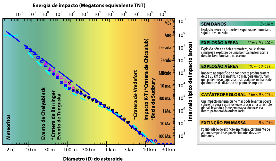
Figura 12. Diagrama da frequência e energia do impacto de objetos com a Terra em função do tamanho do objeto. À direita, resumo dos efeitos esperados para cada classe de impacto. *O local correspondente das indicações dos eventos e crateras na figura representa o diâmetro aproximado dos respectivos asteroides envolvidos; os diâmetros das crateras foram apresentados no texto. Legenda: ma. = milhares de anos; Ma. = milhões de anos. Fonte: modificado de Pierazzo & Artemieva (2012).
