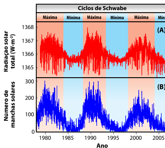
Figura 1. Ciclos de Schwabe – alternância entre períodos de máximas e mínimas solares, conforme exibem as variações (desde 1978) da: (A) radiação solar total e (B) do número de manchas solares. Fonte: modificado de Schöhl et al. (2007).
