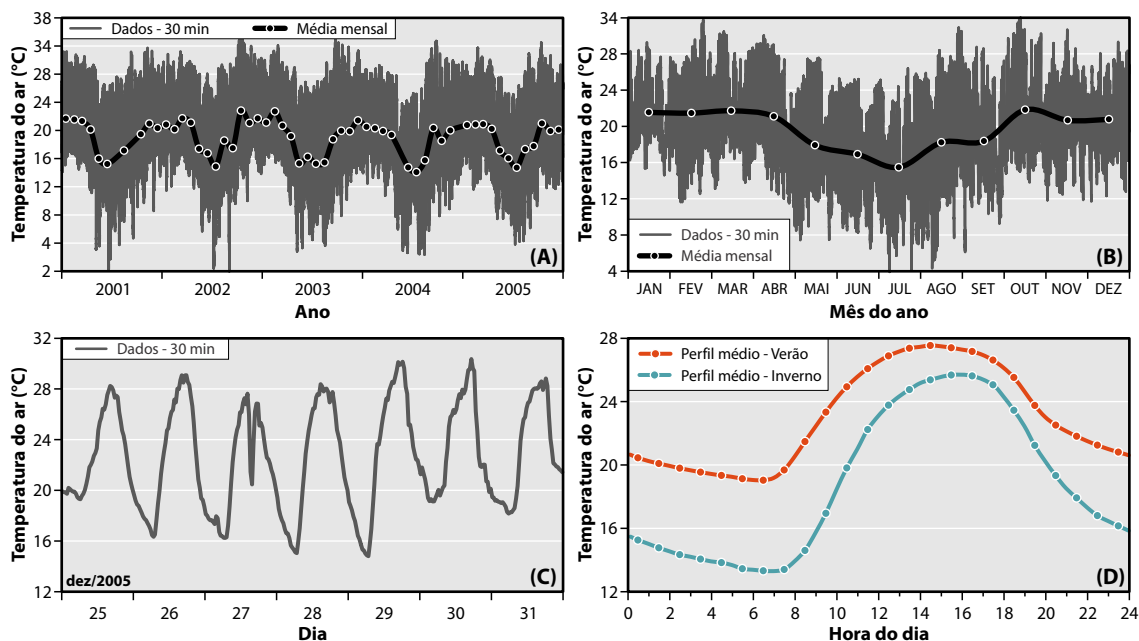
Figura 6. Exemplos de ciclos anuais e diários da temperatura do ar. (A) Cinco ciclos anuais (2001-2005); (B) Um ciclo anual (2005); (C) Sete ciclos diários (25-31 dez/2005); (D) Dois ciclos diários médios provenientes de dados obtidos a cada 30 minutos. Fonte: elaboração própria utilizando dados obtidos na estação climatológica do Centro de Recursos Hídricos e Estudos Ambientais, Escola de Engenharia de São Carlos, Universidade de São Paulo (CRHEA/EESC/USP), Itirapina/SP.
