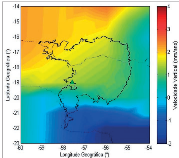
Figura 4 Modelo de V_{up} (componente Up) da Bacia pantaneira, com relação ao bloco norte, alçado a razão de velocidade de 1,5 mm/ano. Em preto, limites da Bacia do Pantanal.
