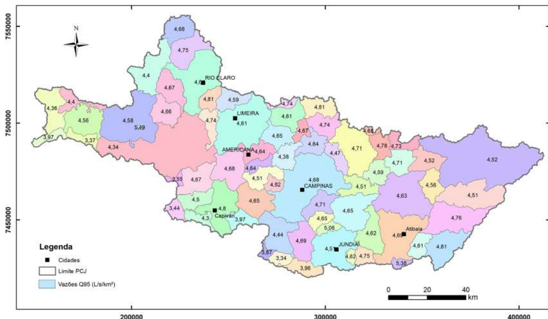
FIGURA 3 – Vazões mínimas Q_{95} (L/s/km 2 ) das Bacias PCJ.
